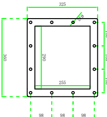
4-72-3.6 出风口 厚度3.0
